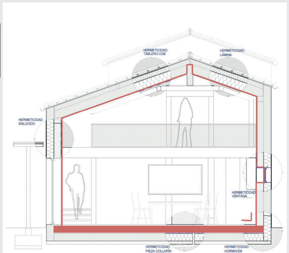
(figura 3) Hermeticidad. Fuente: Propiedad. Passivhaus Consultores. Autor VAND arquitectura
