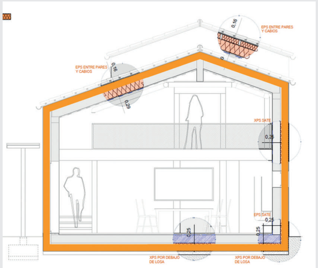
(figura 2) Aislamiento Fuente: Propiedad. Passivhaus Consultores. Autor VAND arquitectura
